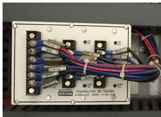
Transdutor de tensão Kron carga 0-750 OHMS
