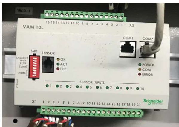
Relé de Proteção p/arcos elétricos VAM 102 Schneider
