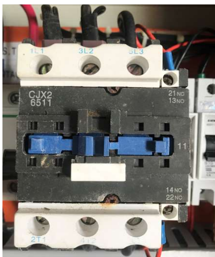
Contatora JNG CJX2-6511
