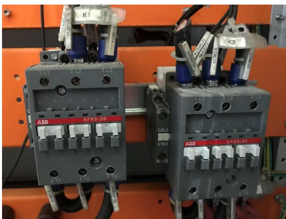
Contatora ABB AF63 30
