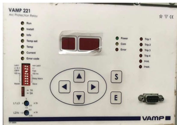
Relé de proteção Schneider Vamp 221
